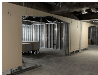
▲1階石膏ボード施工
